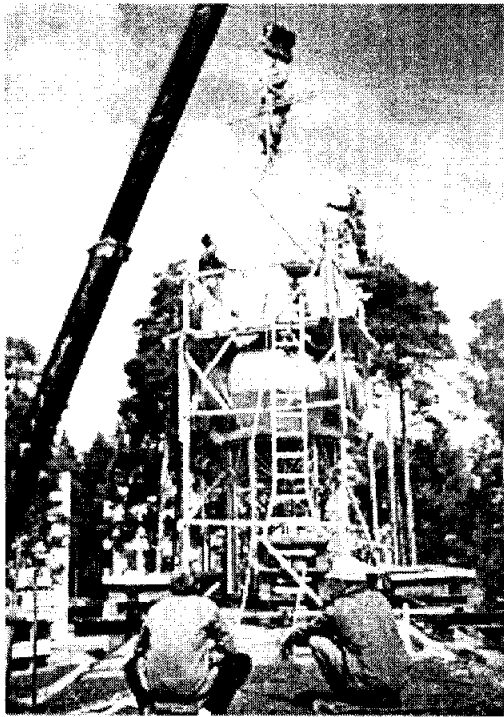
Установка купола на храм Рождества Иоанна Предтечи
